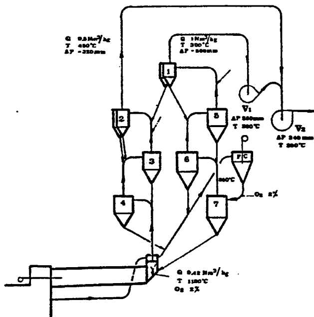
Separate-line calciner
